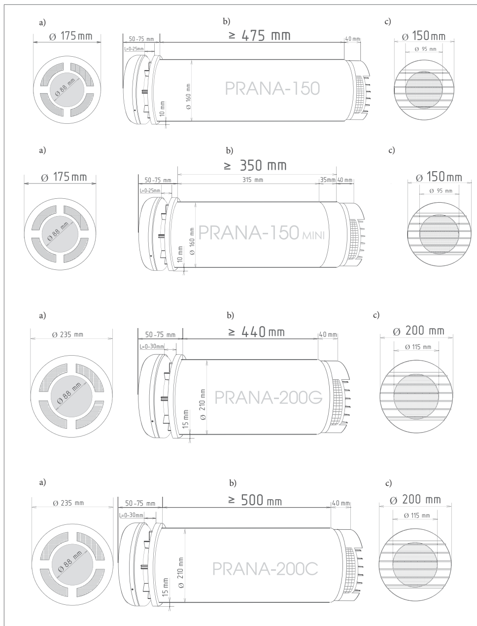
Рис. 3. Габарити і розміри системи вентиляції «PRANA-150», «PRANA-200G», «PRANA-200C»: а) вентиляційна решітка і повітрязабірник у приміщенні; б) моноблок, вигляд збоку; с) вентиляційна решітка і повітрязабірник з вулиці.
